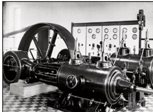
Parný stroj Českomoravská - Kolben z roku 1924
